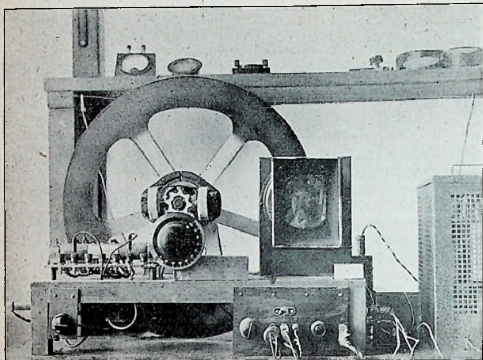
Fig. 6. De televisior met het in 't vorig No. beschreven klemmenbordje rechts onder het beeldvenster.
